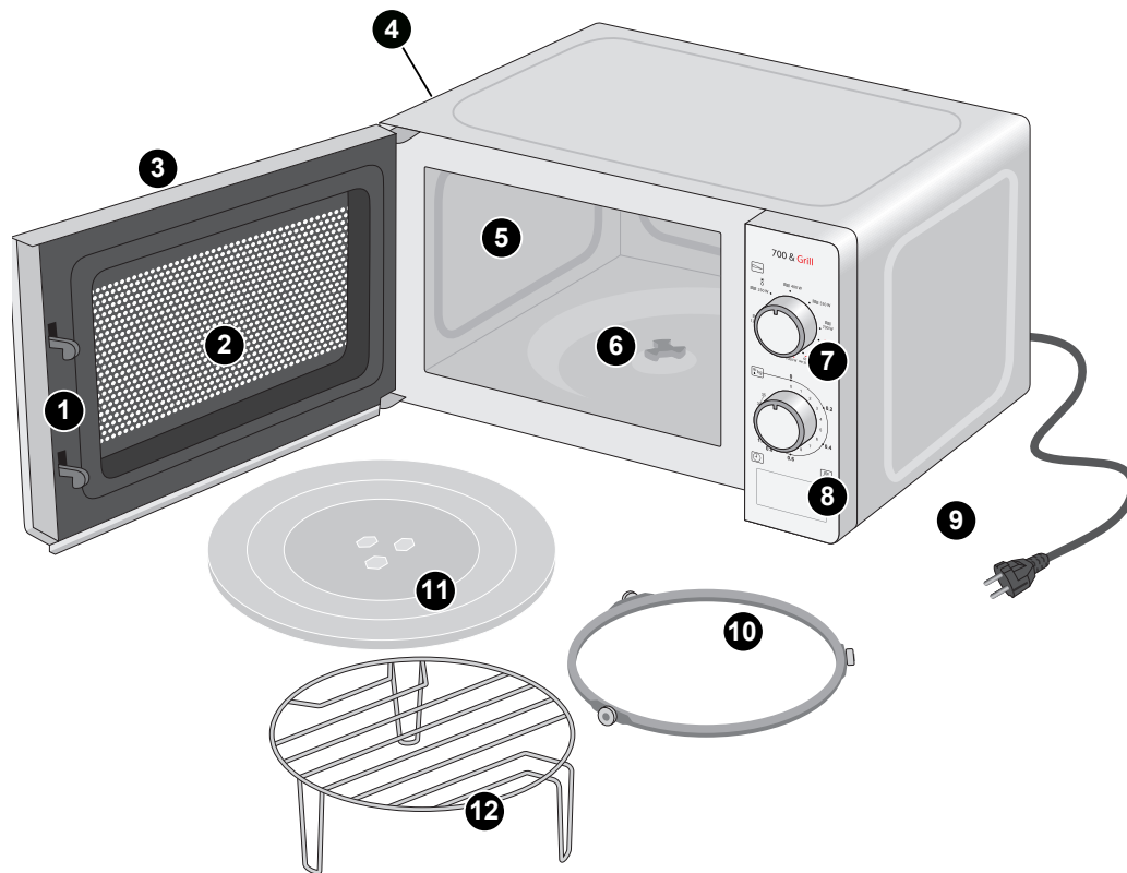
Afb. 1: Onderdelen van het apparaat
